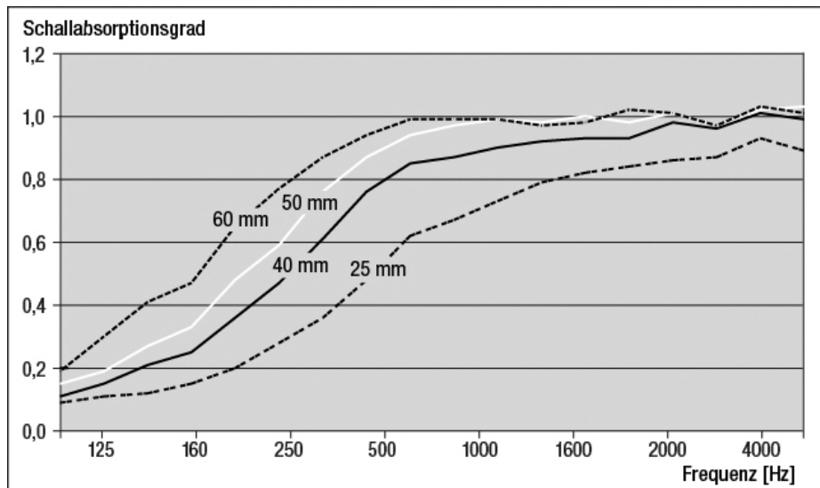
Diagramm 3: Schallabsorptionsgrad von Basotect® B in Abhängigkeit von der Dicke nach DIN EN ISO 354 (Hallraum)
